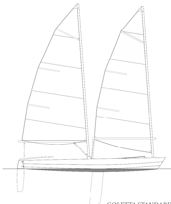
GOLETTA STANDARD
